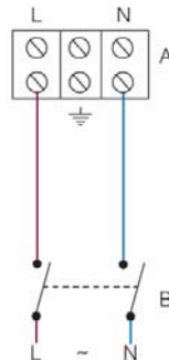
B - Dvojpolový vypínač
